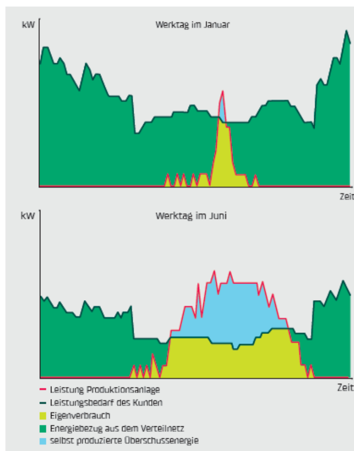
Abbildung 1: Eigenverbrauch an einem Winter- und Sommertag.
